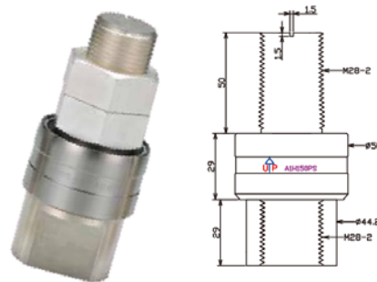
A1H150PS 1pole 1500A
